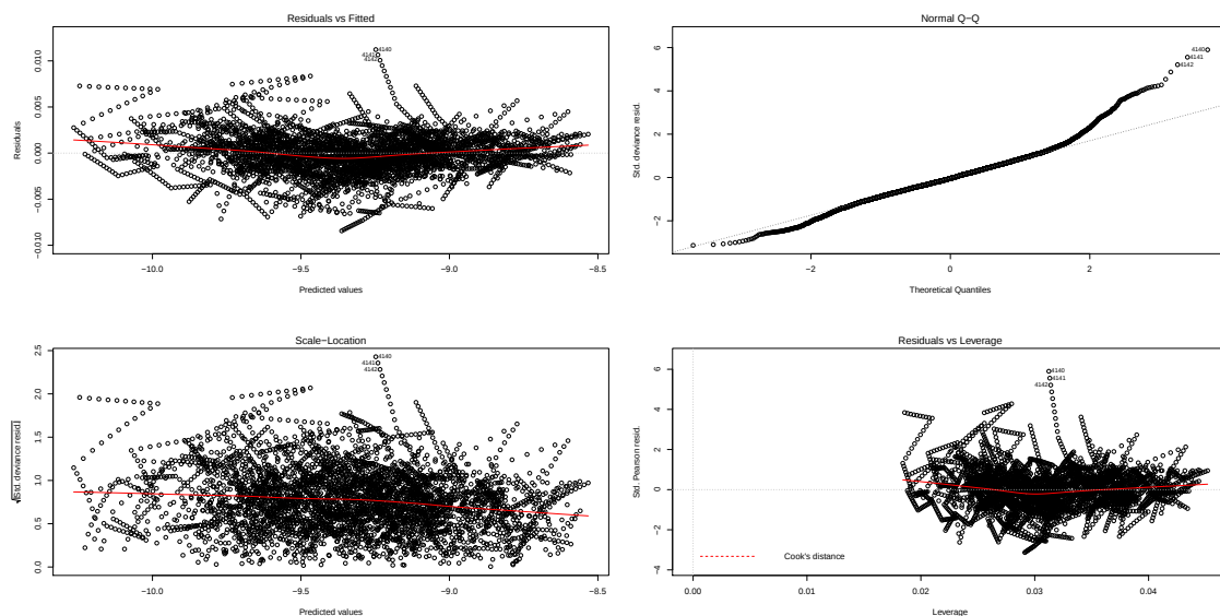
Figure 3: Residuos deviance del modelo para tasa de suicidio (estandarizada) de la población total
