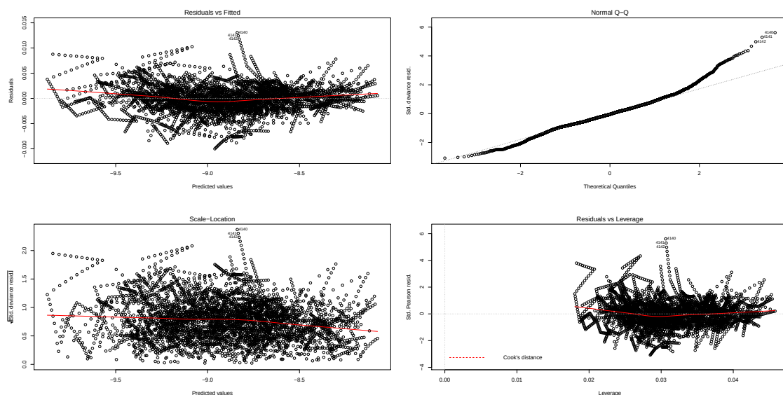
Figure 4: Residuos deviance del modelo para tasa de suicidio (estandarizada) de los hombres
