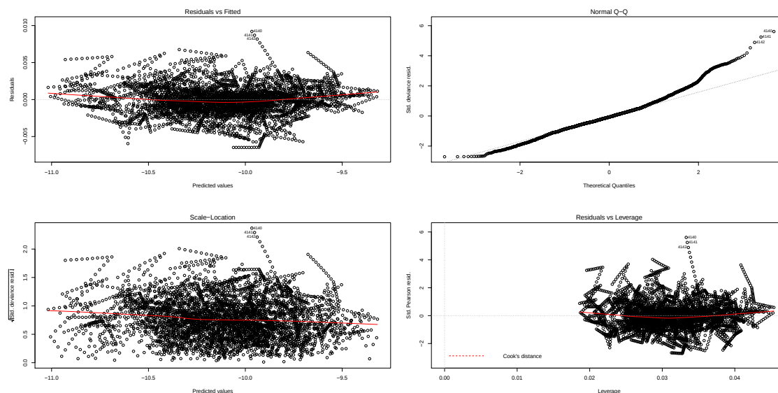
Figure 5: Residuos deviance del modelo para Tasa de suicidio (estandarizada) de las mujeres
