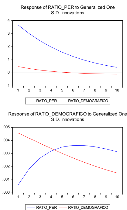
Gráfico 2. Función impulso-respuesta
